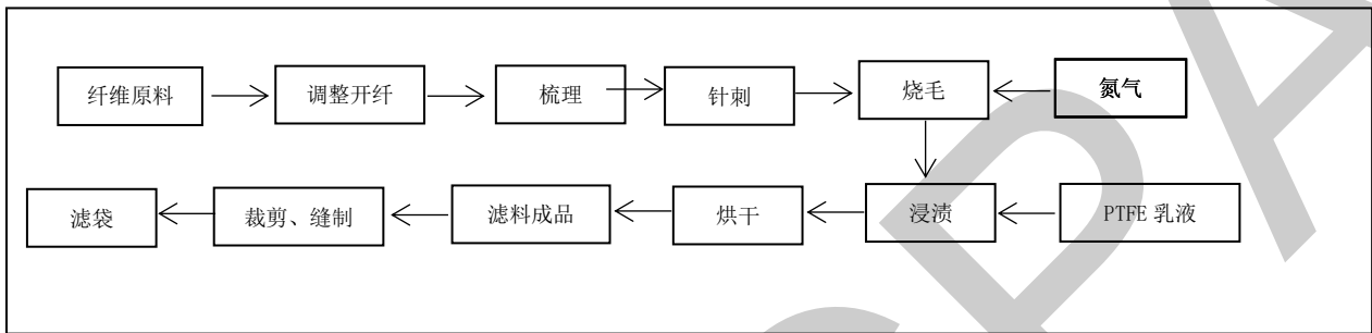
图 A.1 滤袋生产典型工艺流程
