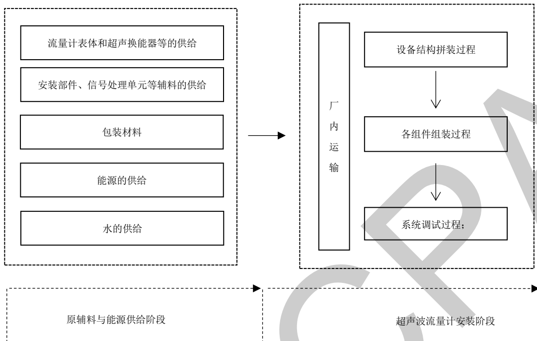
图 1 超声波流量计生命周期系统边界图
