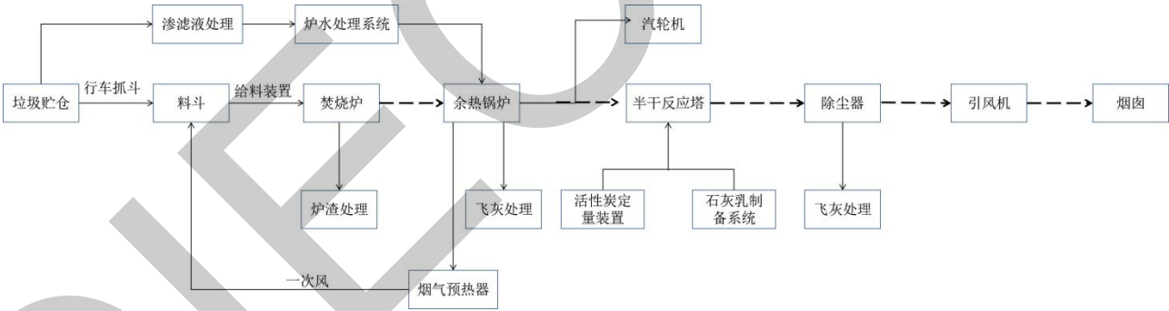
A. 1 垃圾焚烧发电典型工艺流程图
