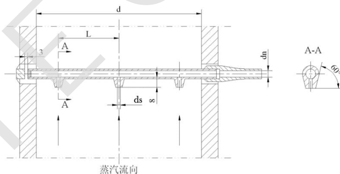
图 B.1 饱和蒸汽采样头
