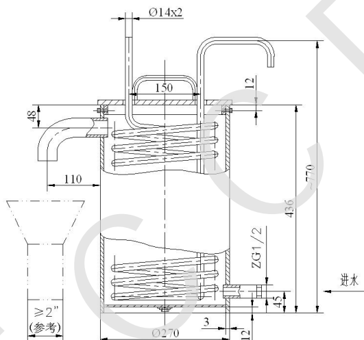
图 B.3 采样冷却器
