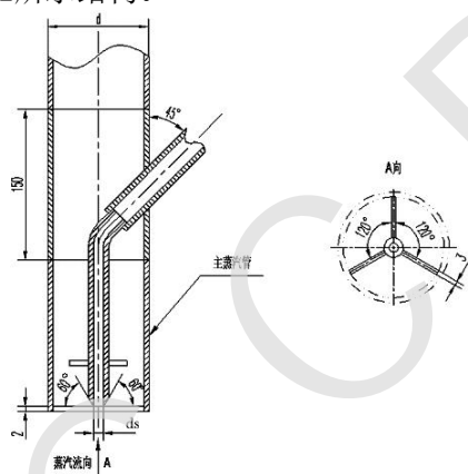
图 B.1 饱和蒸汽采样头
