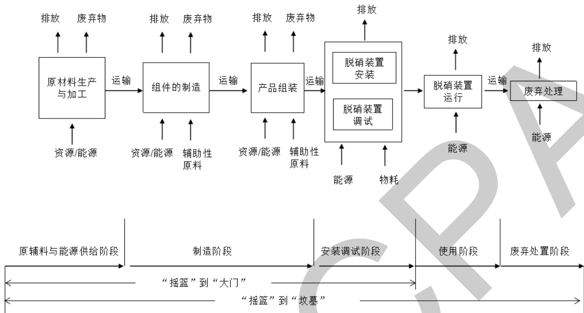
图 1 水泥窑脱硝装置生命周期系统边界
